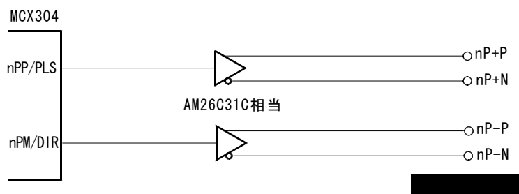
ドライブパルス出力信号回路
