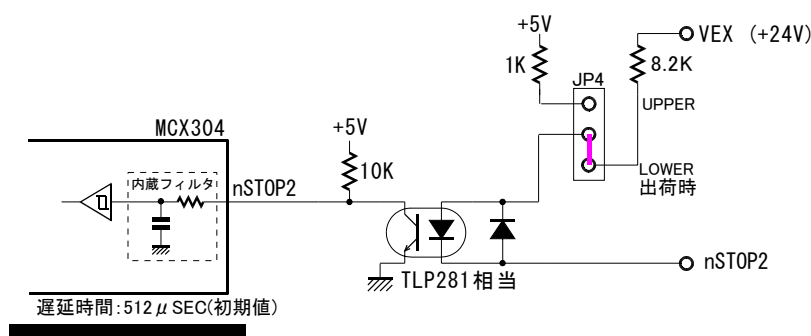
エンコーダZ相入力信号回路
