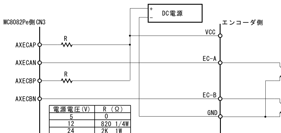
オープンコレクタ出力との接続例
