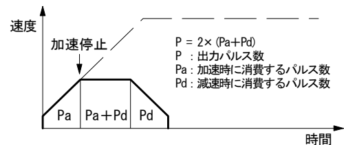
図 2.10 直線加減速ドライブの三角防止
