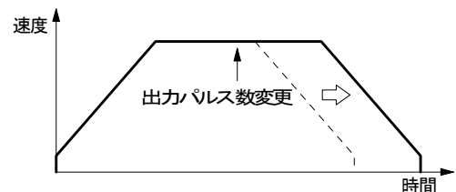
図 2.2 ドライブ途中の出力パルス数変更
