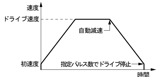
図 2.1 定量パルスドライブ
