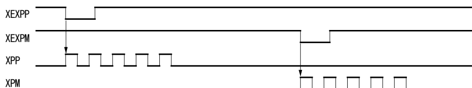
図 2.12-1 外部操作信号による移動パルス数5のX軸相対位置ドライブの例
