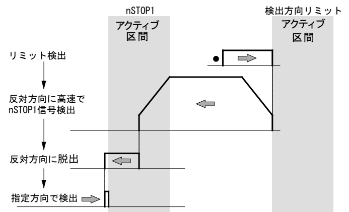
図 2.5-7 ステップ2 イレギュラー動作③
