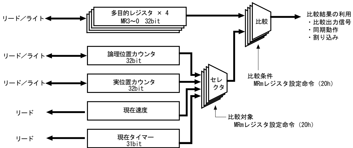
図 2.4-1 多目的レジスタと比較機能
