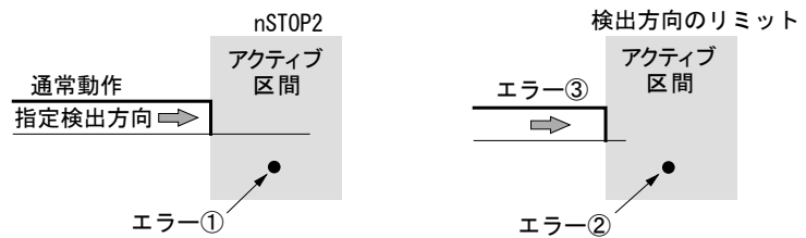
図 2.5-9 ステップ3の動作
