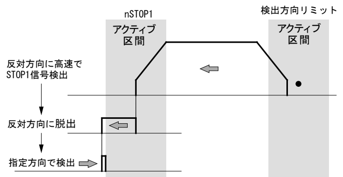
図 2.5-6 ステップ2 イレギュラー動作②
