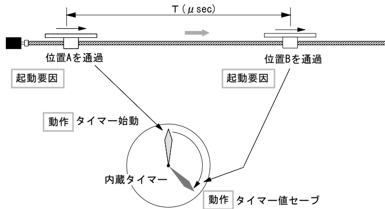
図 2.6-4 同期動作 例4
