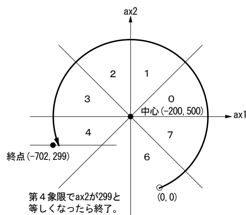
図 3. 2-5 円弧補間終了判定の例
