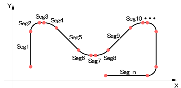
図 1.1-1 連続補間の例
