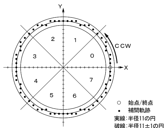
図 3. 2-3 円弧補間例
