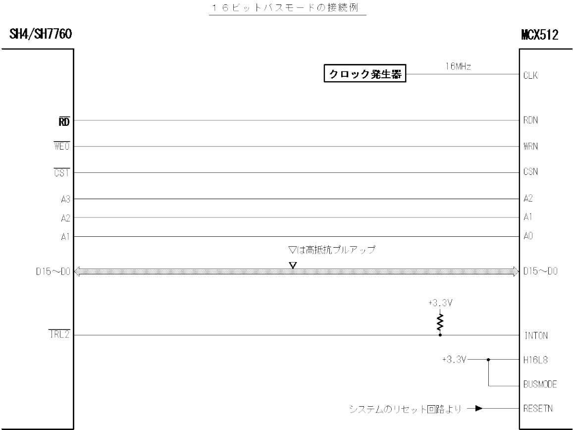
SH-4/SH7760 ウェイト制御例
